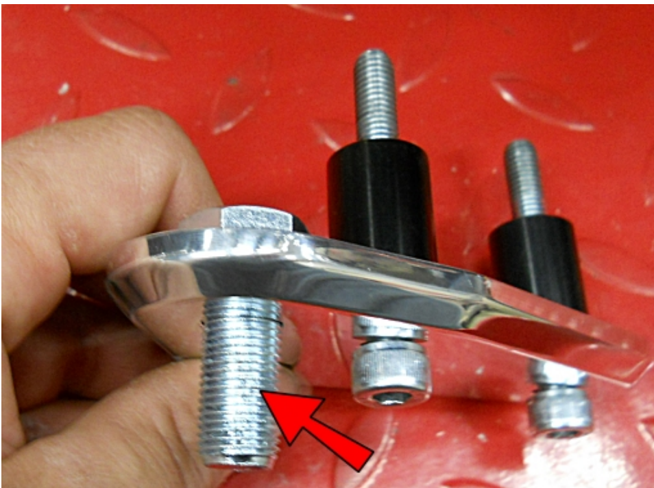
Insert a foot peg bolt.
